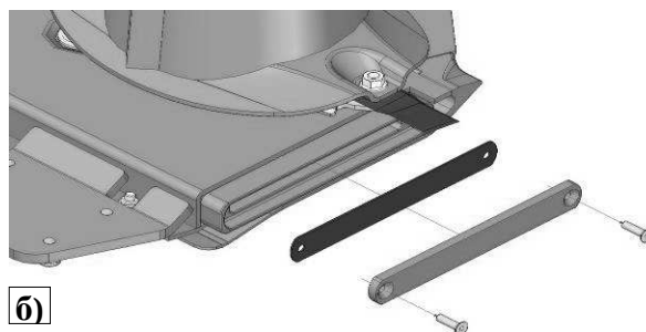
Рис. 31. Пункт контроля а) а также способ смены масла в режущем бруске б)
