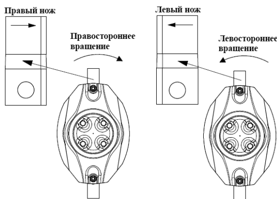
Рис. 17. Схема монтажа режущих ножей
