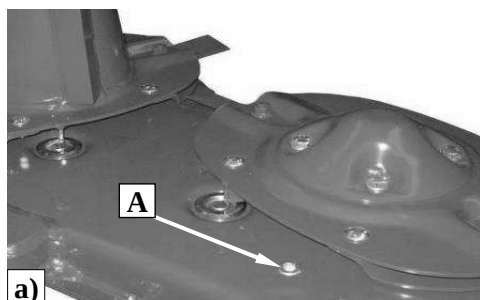
Рис. 31. Пункт контроля а) а также способ смены масла в режущем бруске б)
