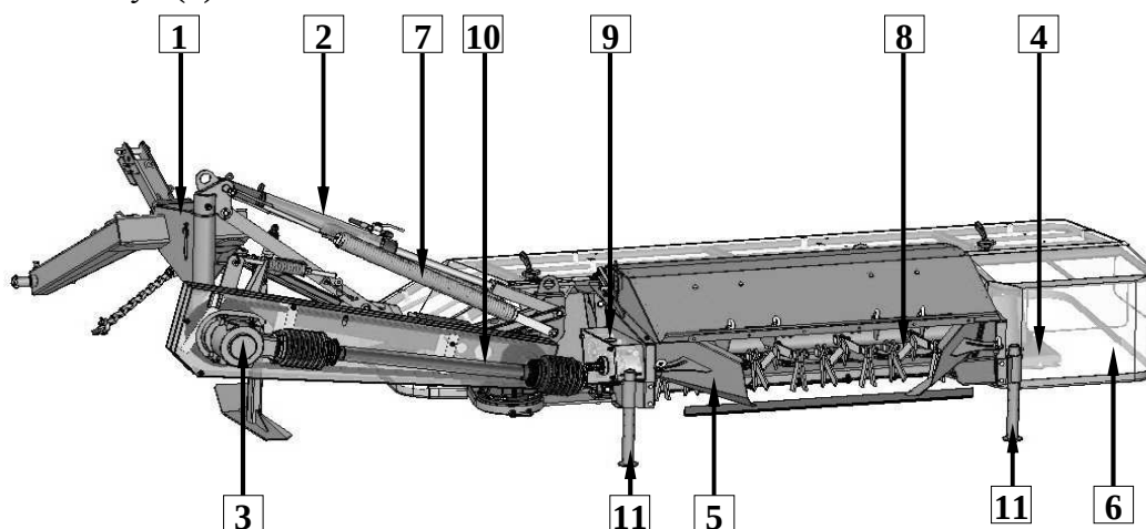
Рис. 3б. Навесная дисковая косилка со вспушивателем
