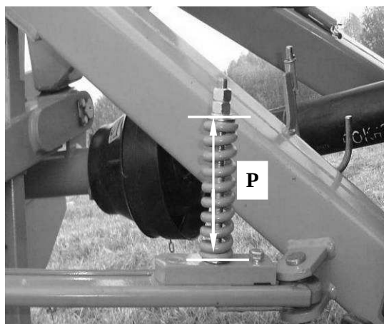
Рис. 14. Тяговый предохранитель косилки
