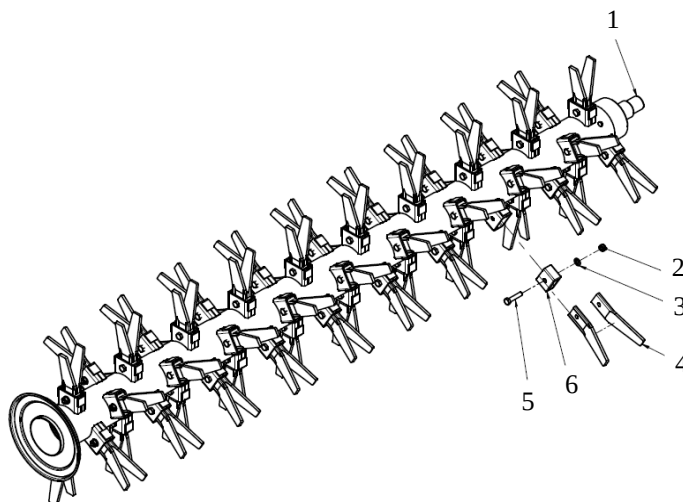
Рис. 26а. Замена битеров впусивателя
