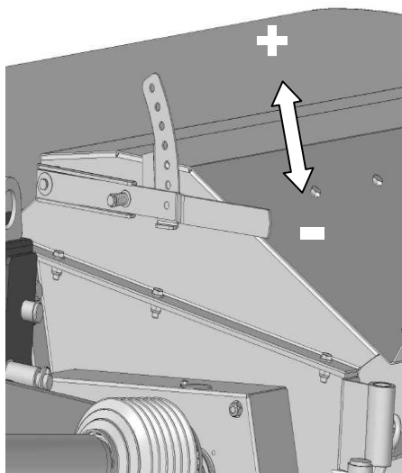
Рис. 25. Регулирование заслонки впусивателя
