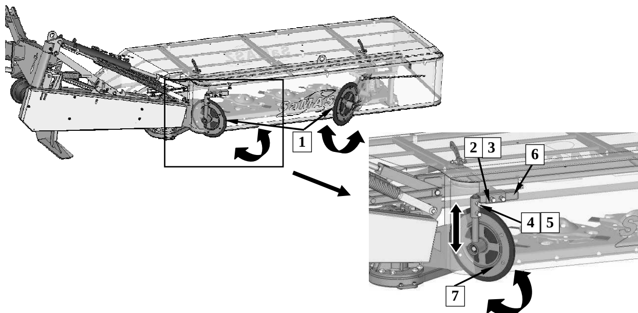
Рис. 19. Регулировка скребков покоса: 1- скребок покоса, 2 – контрящие гайки, 3 – болты регулировки плеча, 4 – контрящие гайки, 5 – болты регулировки диска, 6 – плечо скребка, 7 – диск
