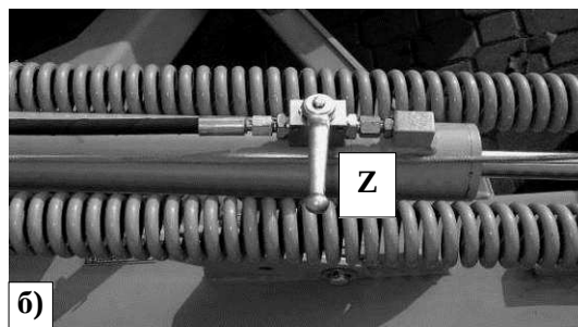
Рис. 10. Положение запорного гидравлического крана гидросистемы: а) открыт О (работа), б) закрыт З (транспортировка)
