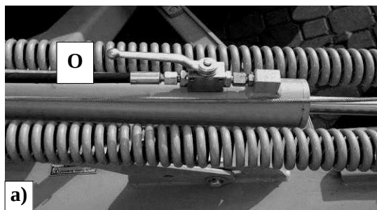
Рис. 10. Положение запорного гидравлического крана гидросистемы: а) открыт О (работа), б) закрыт З (транспортировка)
