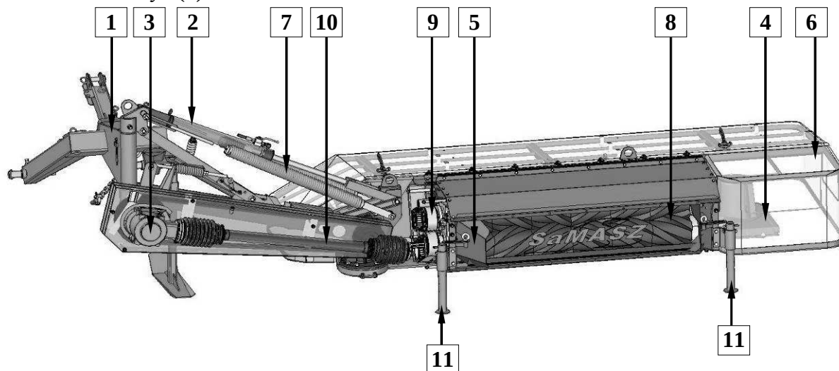
Рис. 3в. Косилка-плющилка навесная дисковая
