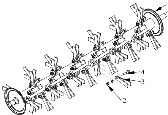
Рис. 26а. Замена битеров впусивателя
