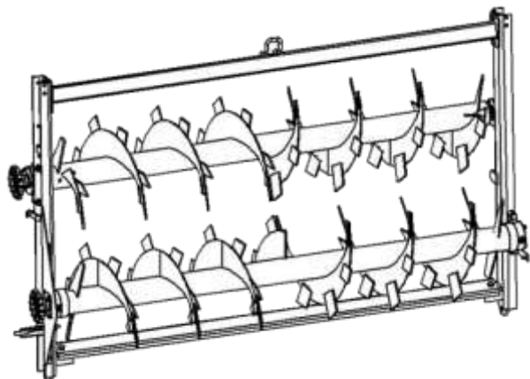
A2HS - 2 горизонтальных шнека Модель N221/4-3
