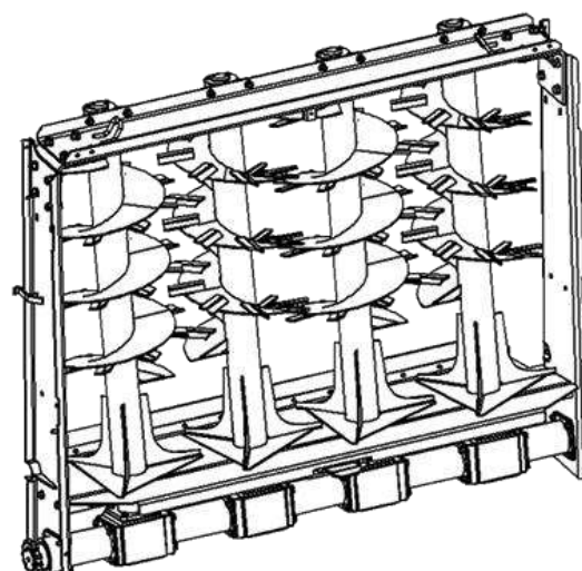
A4VS – 4 вертикальных шнека Модель N221/3-3
